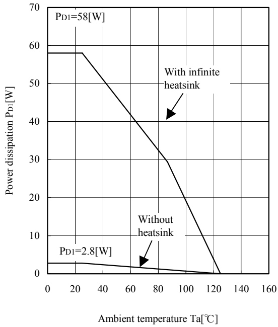
IRIS-F6428S MOSFET Ta-PD1 Curve
